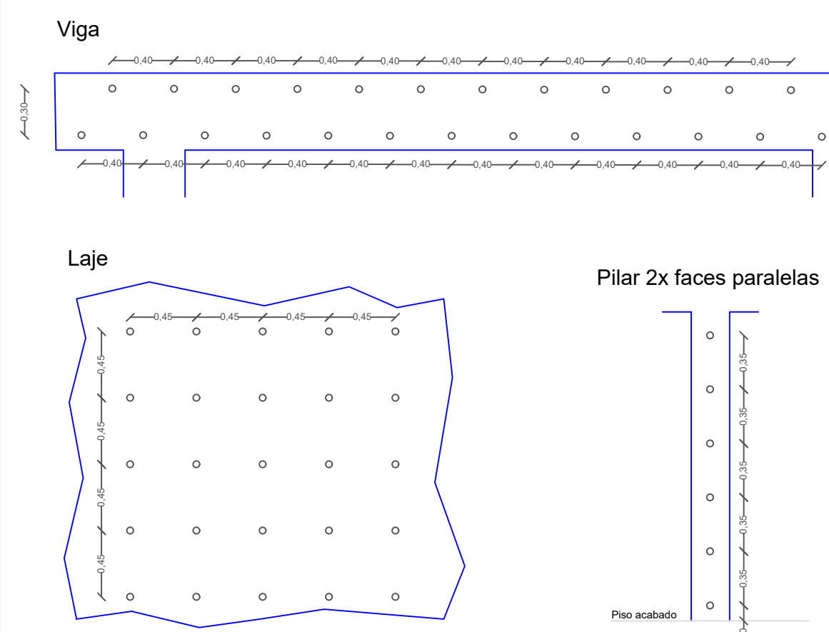
Localização dos furos - Injeção de Realcalinizante Químico
