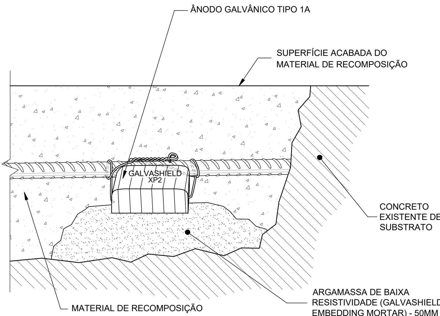
ESQUEMA DE INSTALAÇÃO DETALHE DO ANÓDO GALVÂNICO
