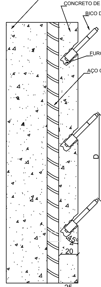
Corte Esquemático - Instalação dos Bicos de Perfuração
